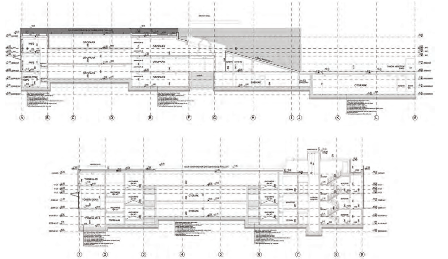
Kesitler
