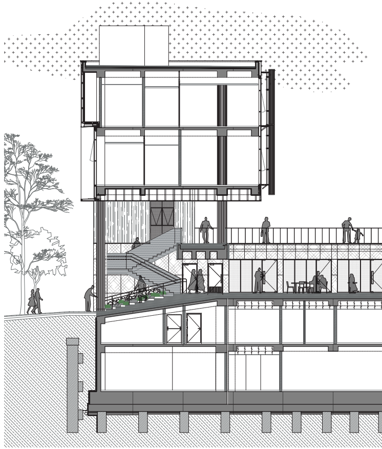
Kesit
