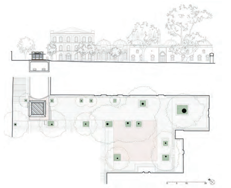
Çınaraltı Vaziyet Planı ve Siluet
