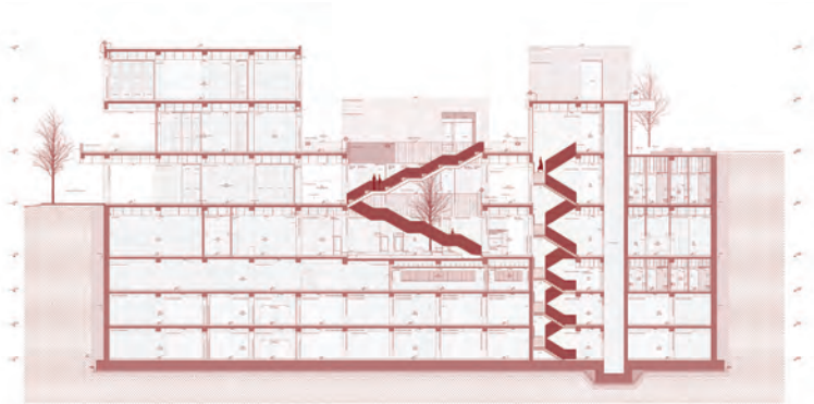
Kesit
