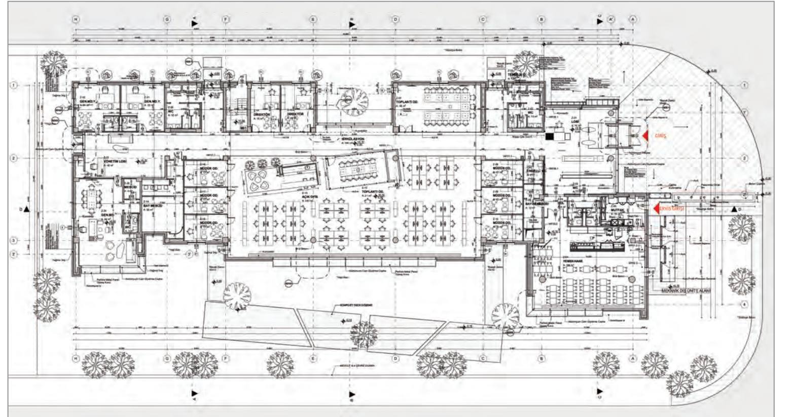
Zemin Kat Planı
