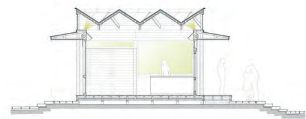
Çınaraltı aa Kesit
